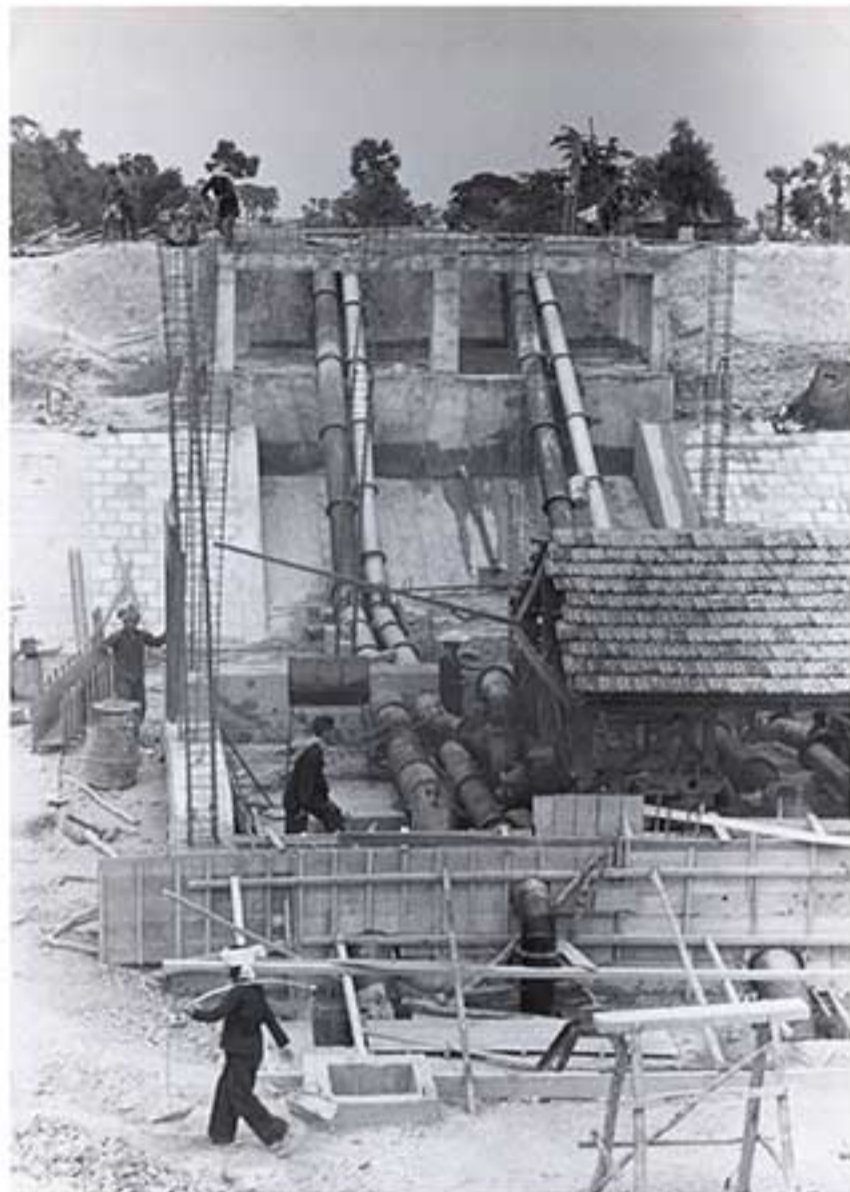
កងកម្លាំងចល័តកំពុងសាងសង់ទំនប់ទឹក Mobile unit workers construct an irrigation
